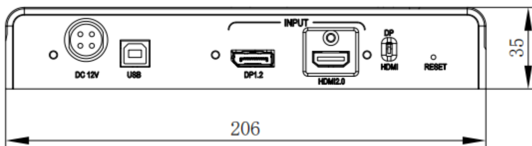
图 3: K0 后视图
