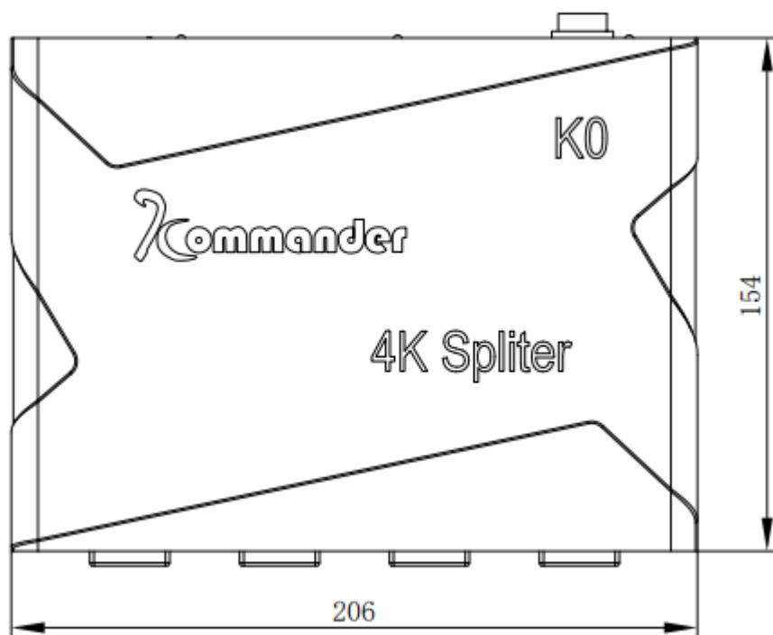
图 1: K0 正视图
