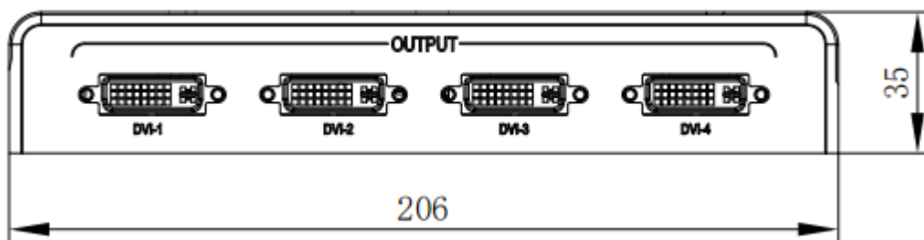
图 2: K0 前视图
